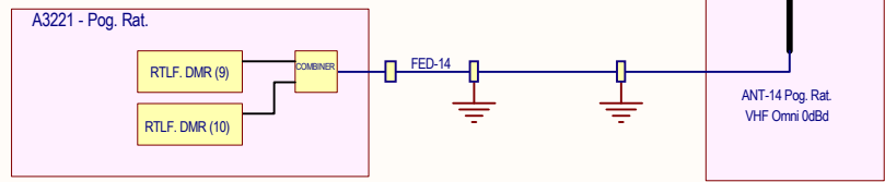
Schemat systemu łączności radiowej - Cz. 1. Rys. 1a
