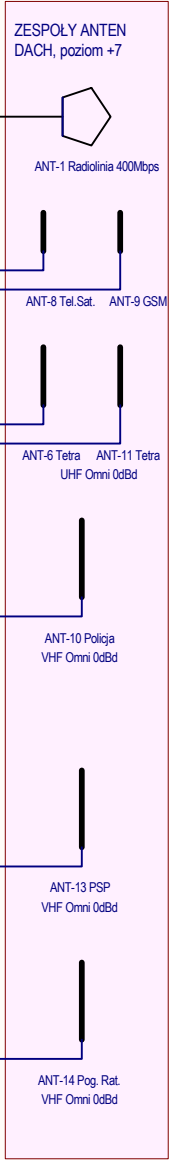
Schemat systemu łączności radiowej - Cz. 1. Rys. 1a
